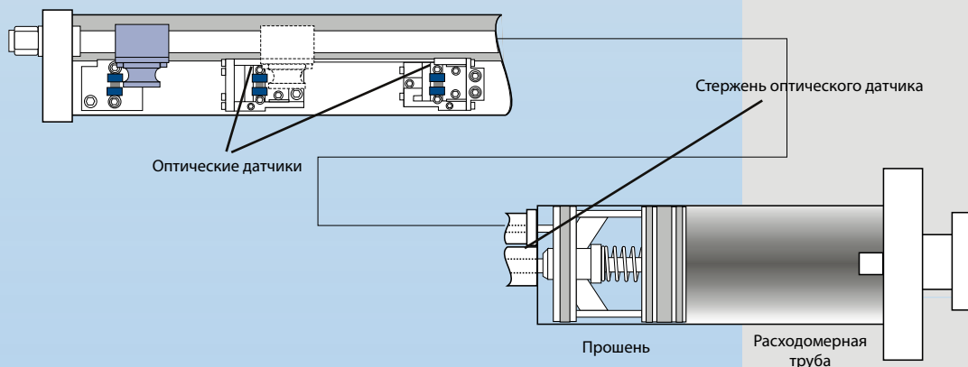
Узел оптического датчика
